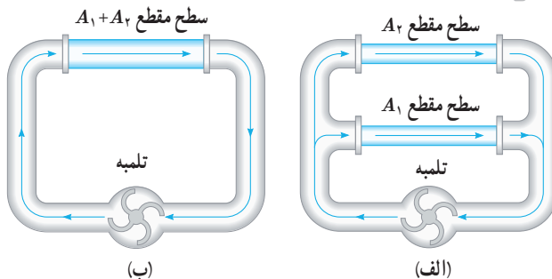
شکل ۲-۴۱ (الف) دو لوله هم طول با سطح مقطع های A_1 و A_2 به طور موازی به تلمبه آبی متصل شده اند. (ب) دو لوله بخش الف معادل با تک لوله ای با همان طول و سطح مقطع مجموع آنهاست.
