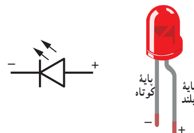
شکل ۲-۲۶ تصویری از یک LED و نماد آن در مدارهای الکتریکی
